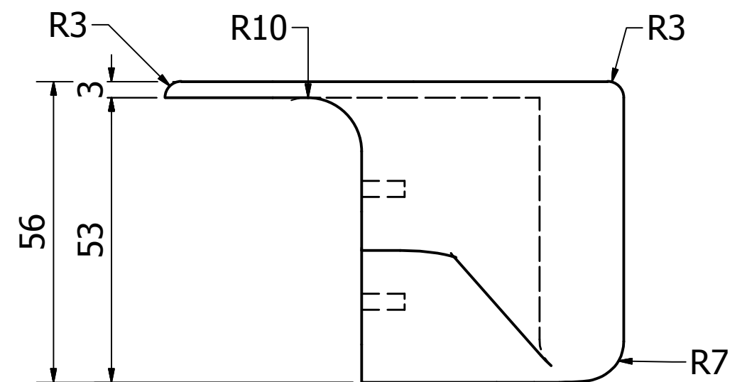
VISTA LATERAL DERECHA
