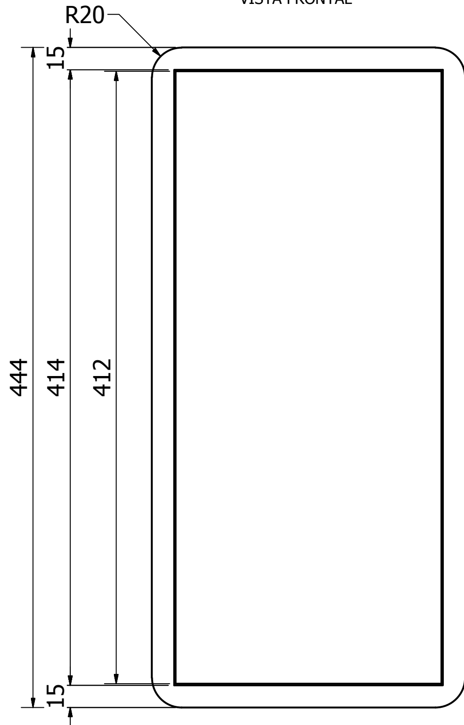
VISTA INFERIOR
