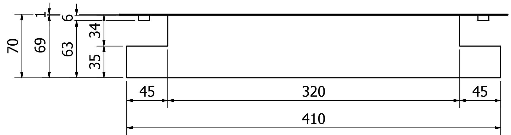
VISTA LATERAL DERECHA
