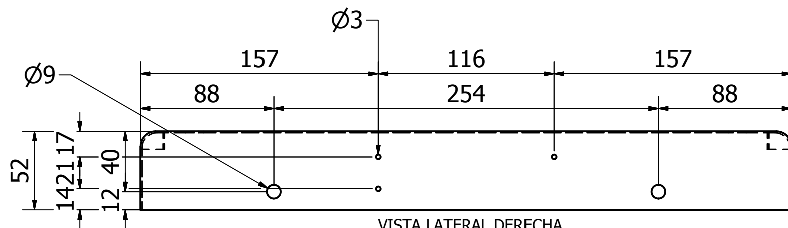
VISTA LATERAL DERECHA
