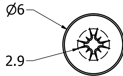
VISTA SUPERIOR
