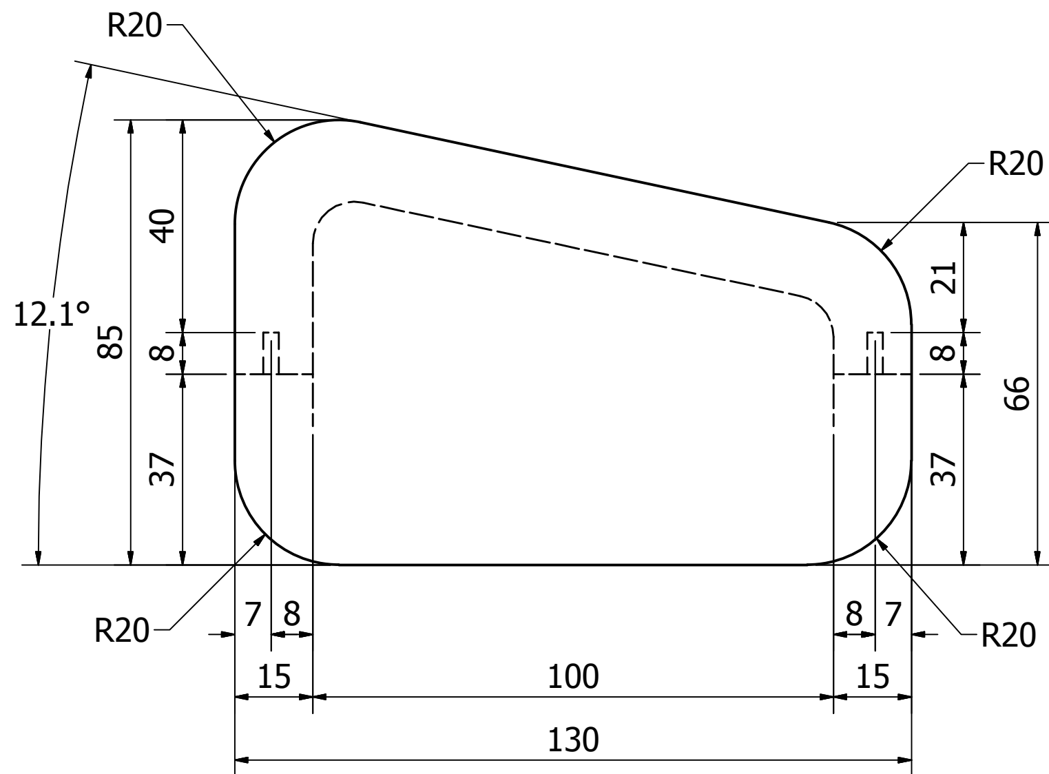
VISTA SUPERIOR
