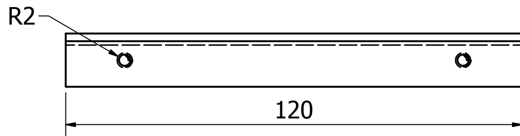
VISTA INFERIOR
