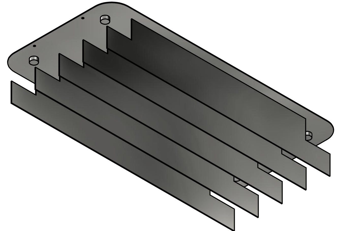
ISOMETRÍA
