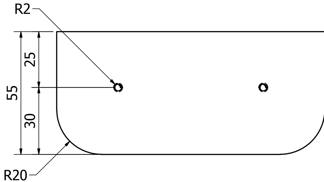
VISTA INFERIOR
