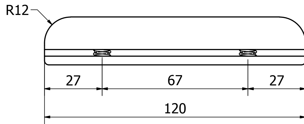
VISTA INFERIOR
