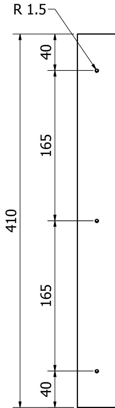
VISTA SUPERIOR
