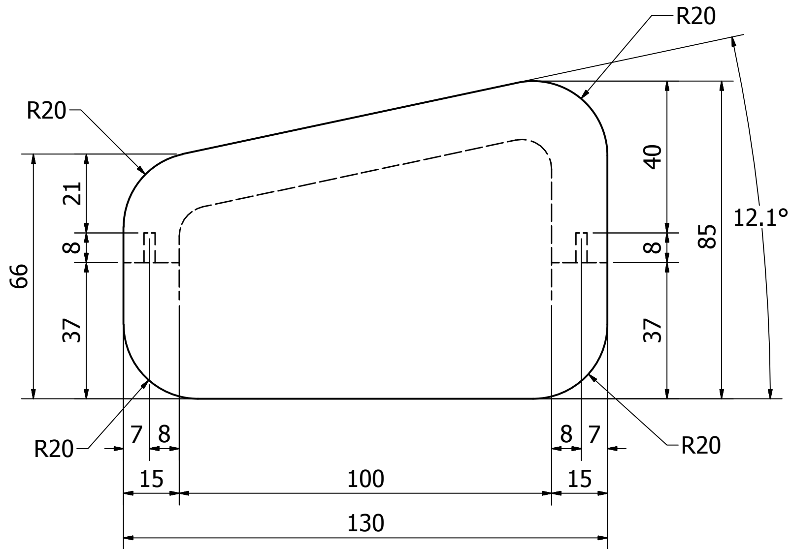
VISTA SUPERIOR
