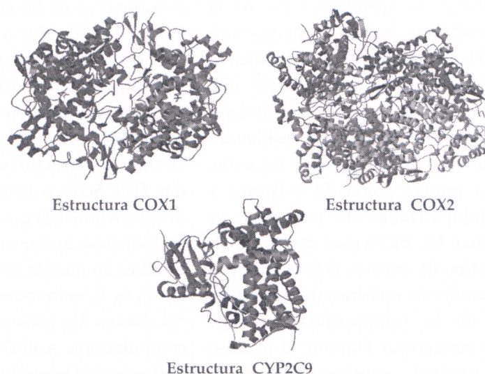
Figura 1. Estructuras de las enzimas Ciclooxygenasa 1 y 2 (COX-1 y COX-2) y citocromo P450 2C9 (CYP2C9) obtenidas de las base de datos Protein Data Banks
