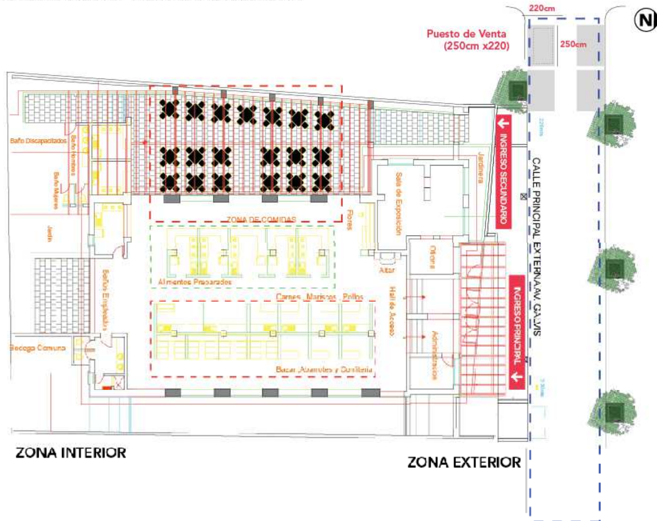
PLANO MERCADO Plano Final Rediseño "Mercado la Floresta" Dirección de Comercialización
