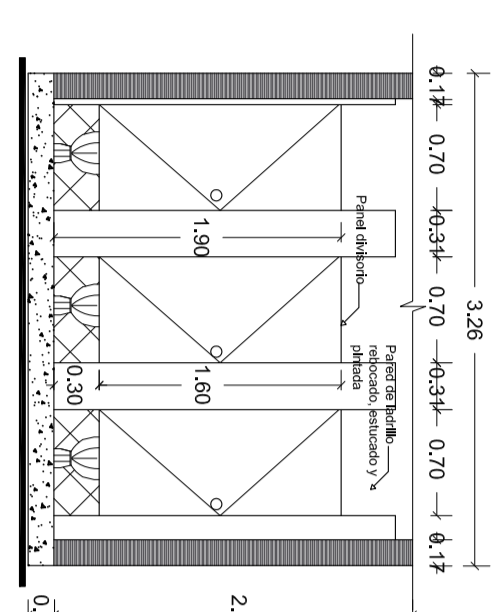
Fachada 3 Esc: 1 ___ 50
