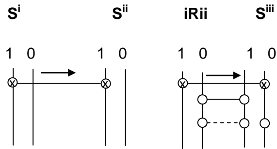
Figura N. 23 Cálculo cuando inicia en Valor para (AxB) \neq C
