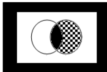
Figura N. 6 Diagrama de Venn para la Concepción Estética Kantiana.
