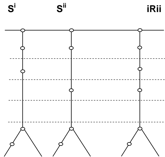
Figura N. 25 Diagramas de Quipus para la Suma Trunca en 1.
