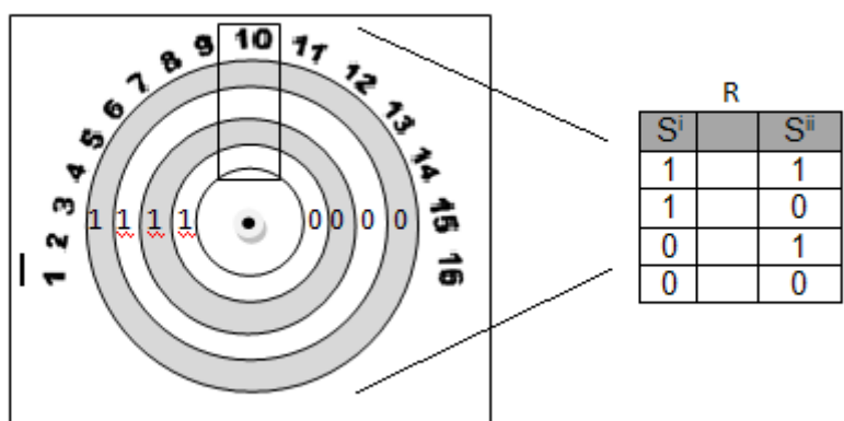
Fig. N. 2 Máquina de Lull para Lógica Monovalente limitada.
