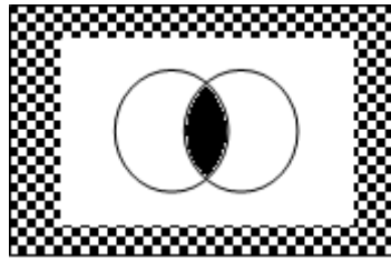
Figura N. 9 Diagrama de Venn para la Multiplicación en Conjunción con la División.
