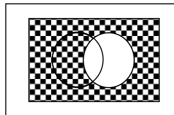
Figura N. 10 Diagrama de Venn para la relación Multiplicación-División en Exclusividad Izquierda.
