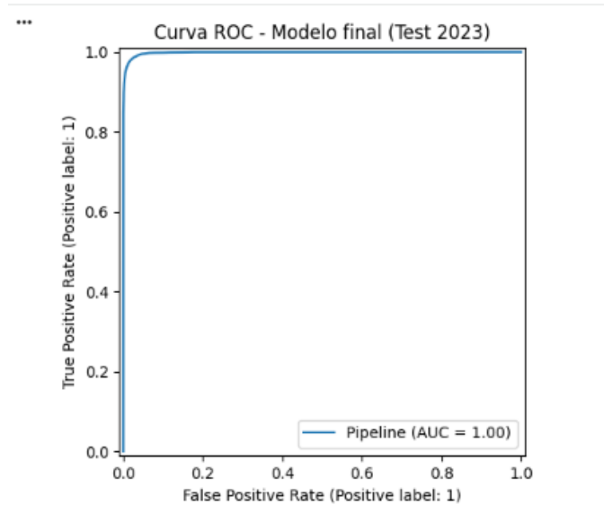
Ilustración 47. Curva ROC-Modelo Final
