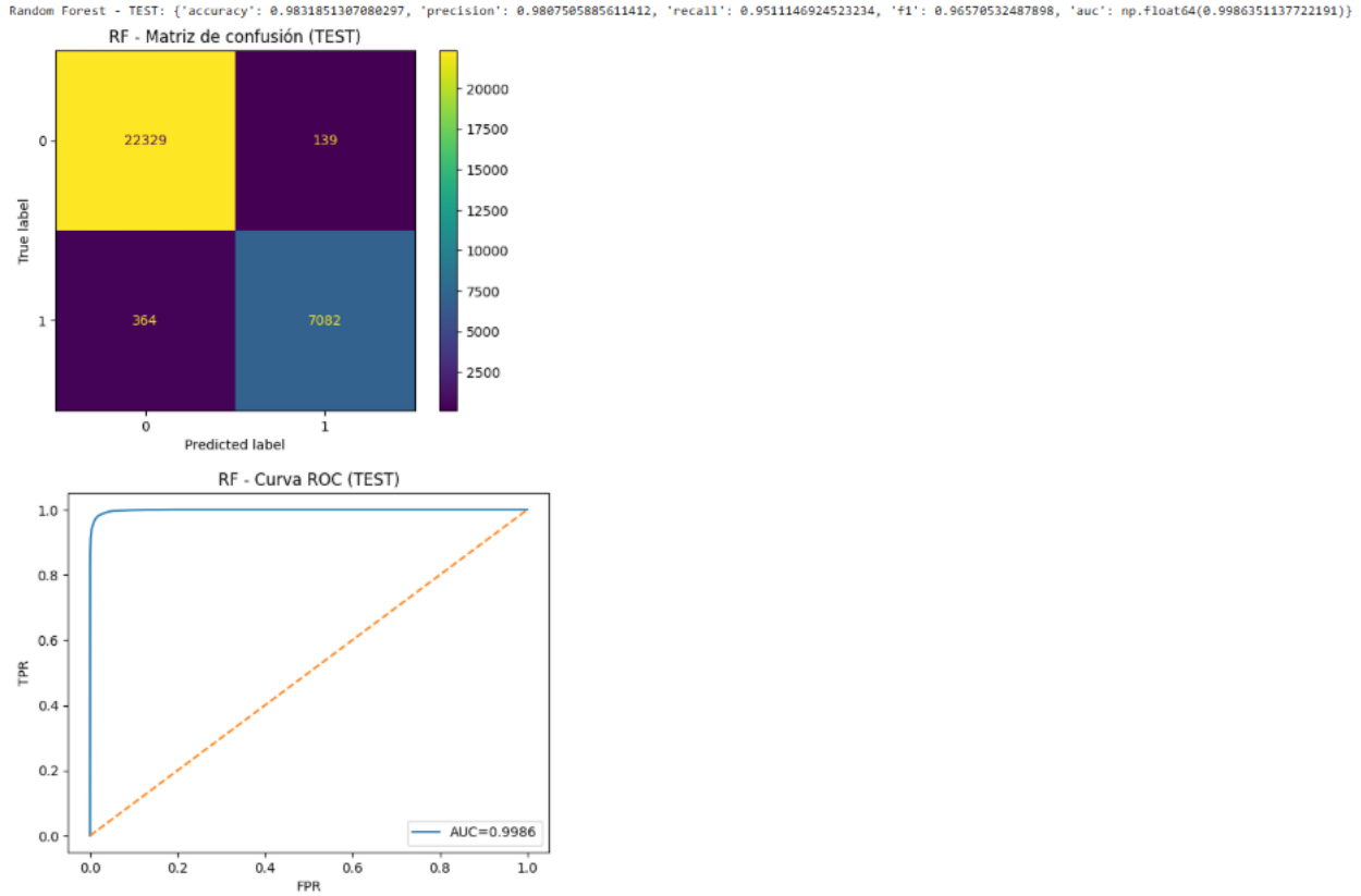
Ilustración 36. Matriz de confusión(TEST)
