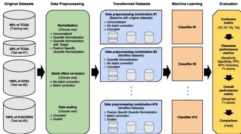
Ilustración 5. Pipeline general de preprocesamiento(ML)
