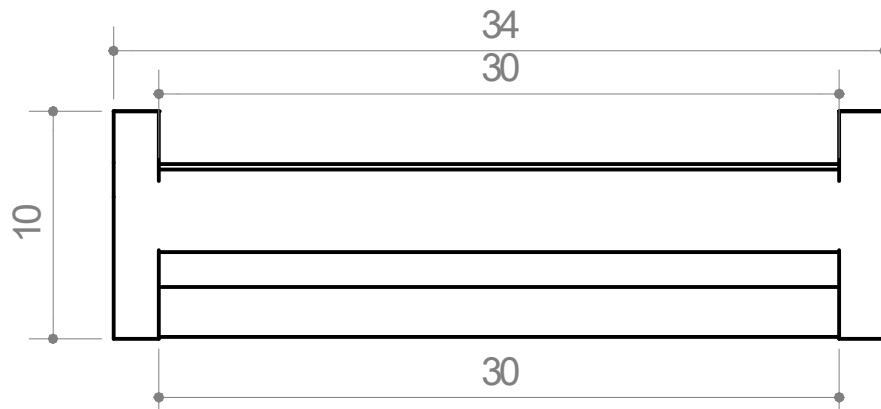
Vista superior
