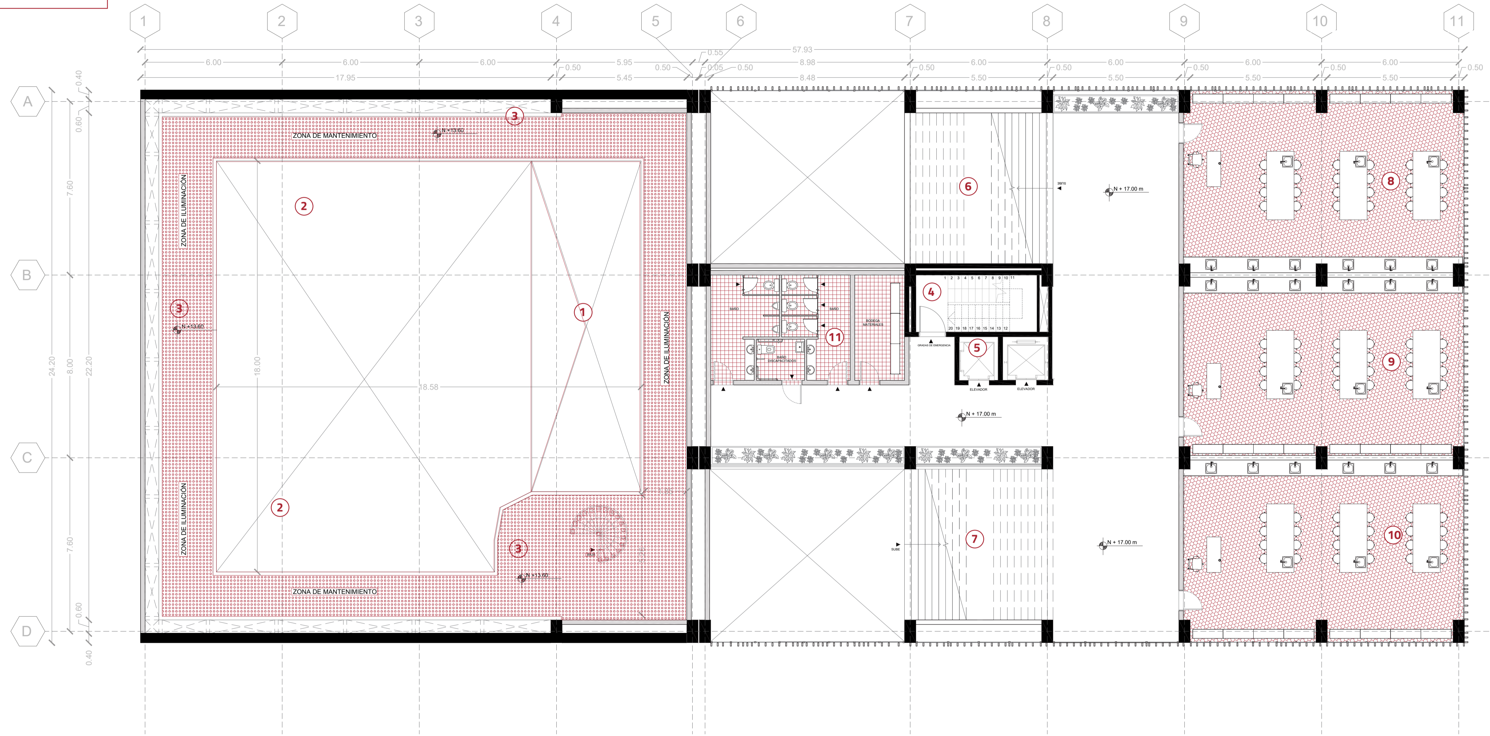
PLANTA AUDITORIO + FÁBRICA TALLERES 2 ESC 1:100 NIVEL + 17.00 m
