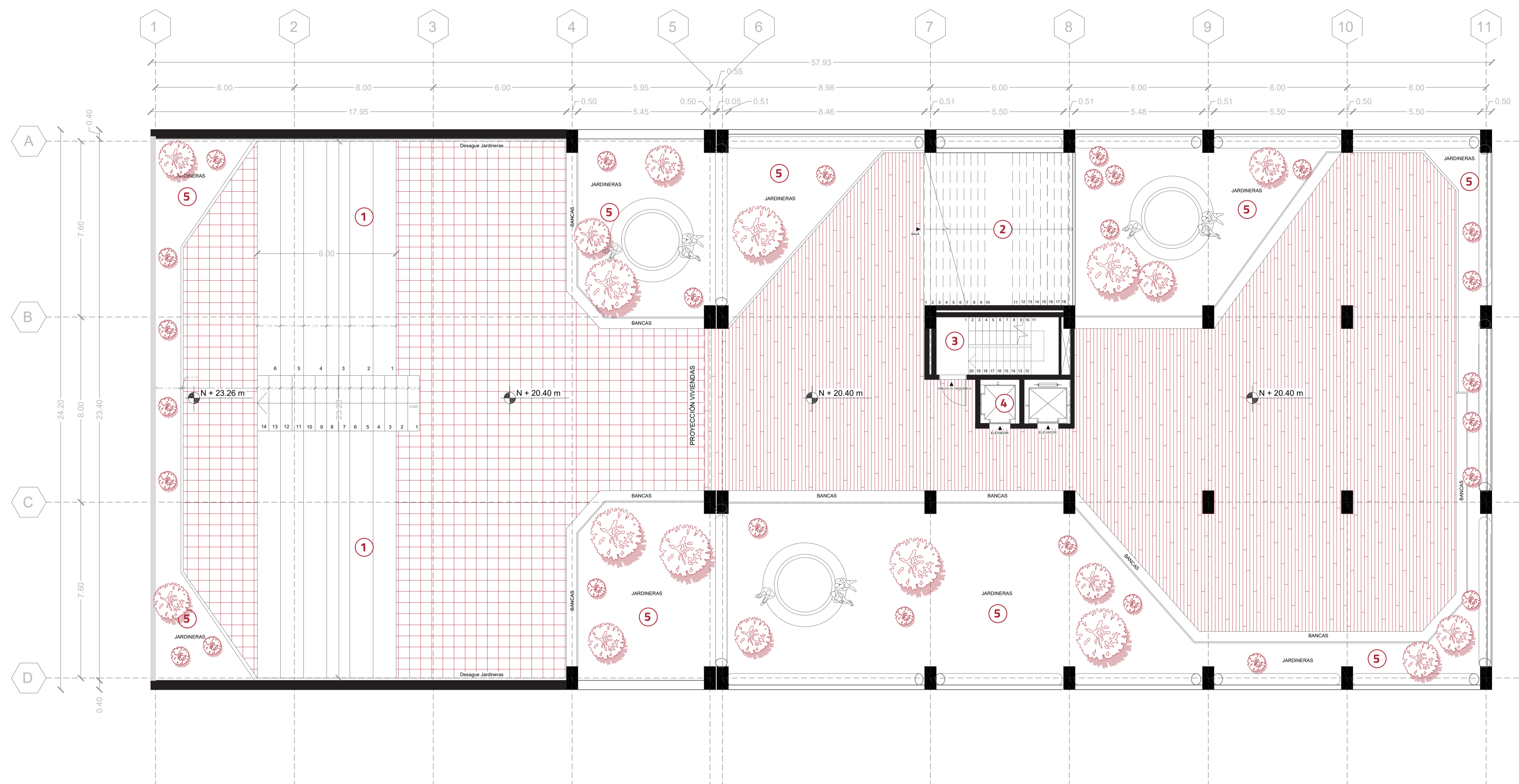
PLANTA TERRAZA COMUNAL 1 ESC 1:100 NIVEL + 20.40 m
