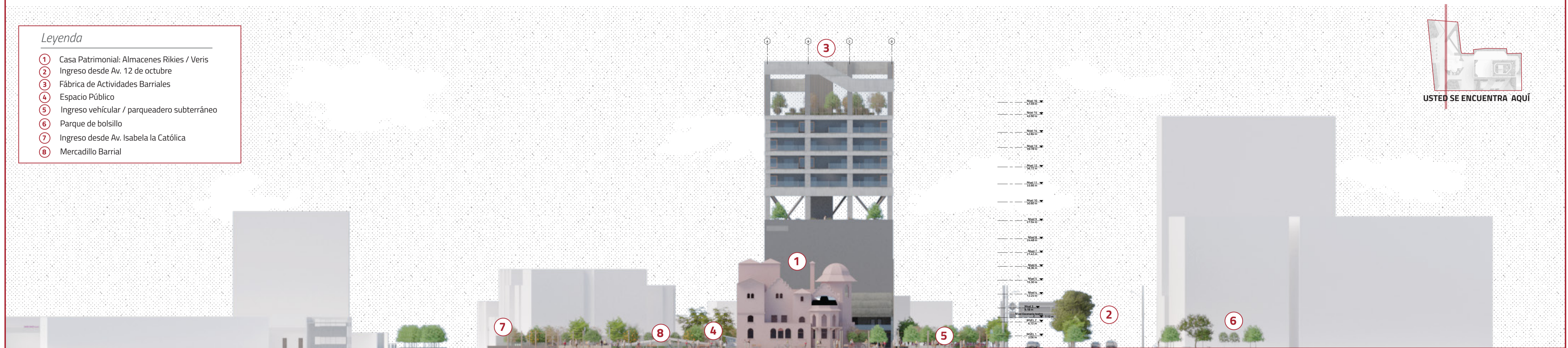
CORTE URBANO 3: FÁBRICA LA FLORESTA ESC 1:500 NIVEL +/- 0.00m
