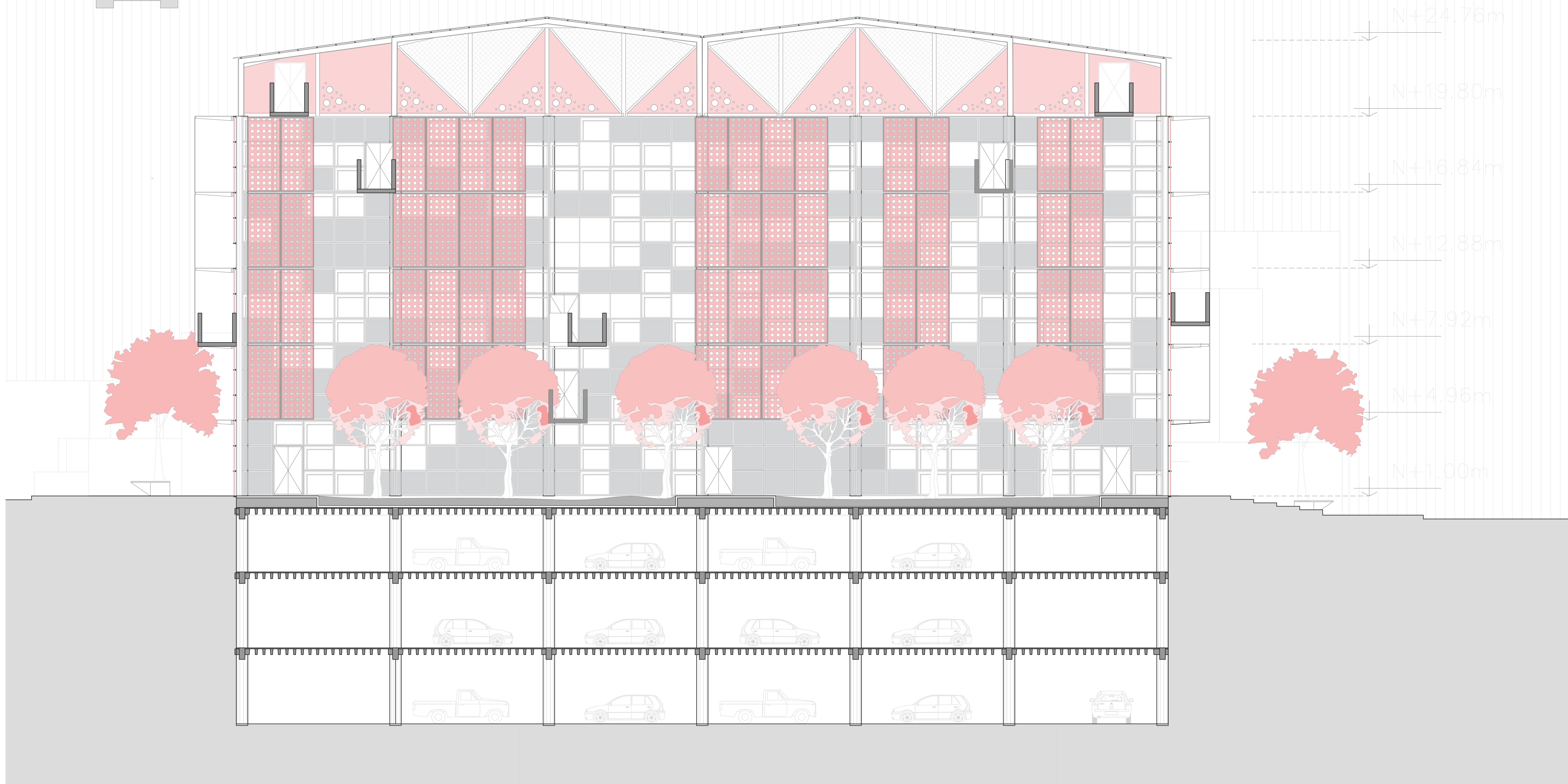
CORTE A-A'
