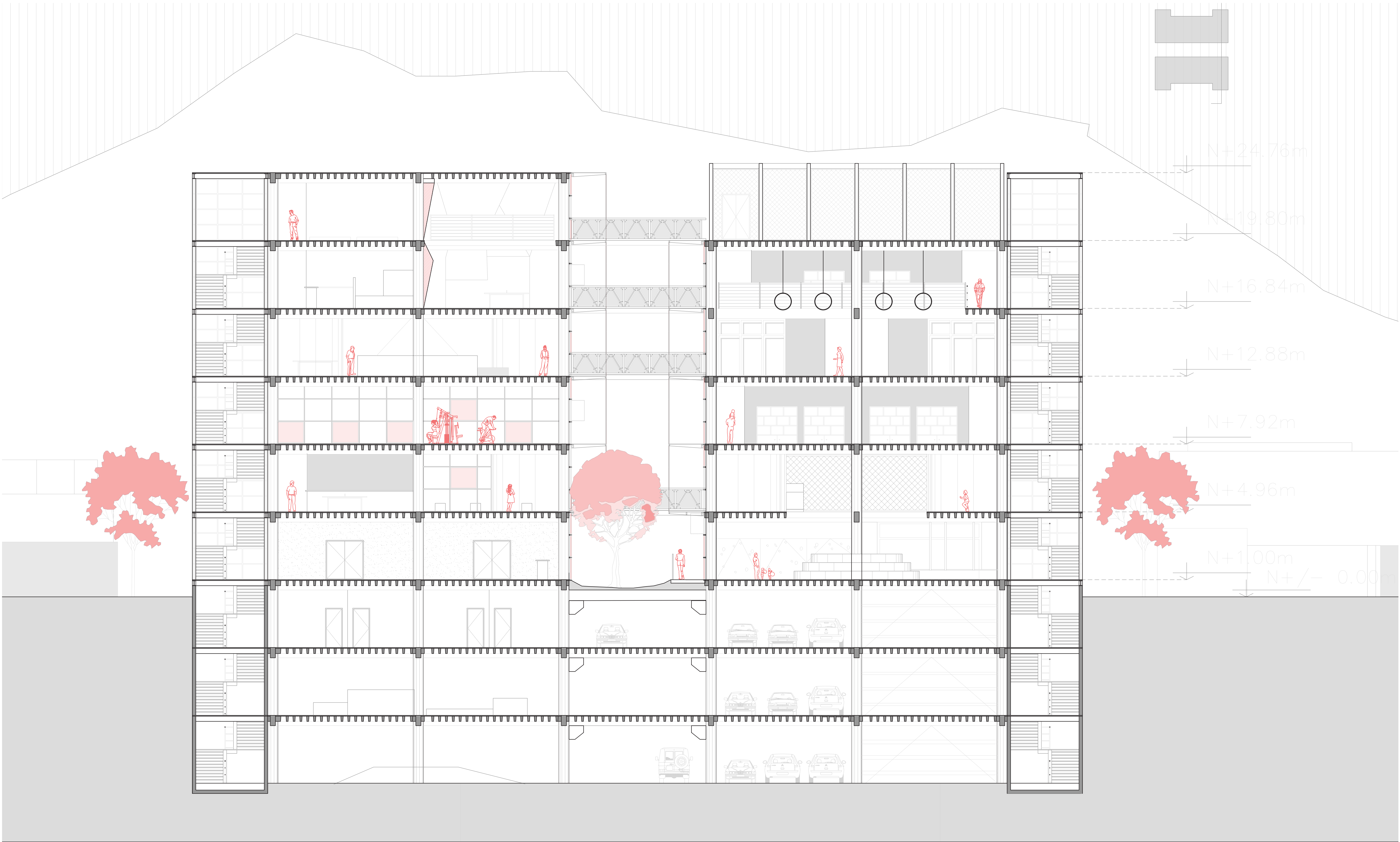
CORTE B-B'
