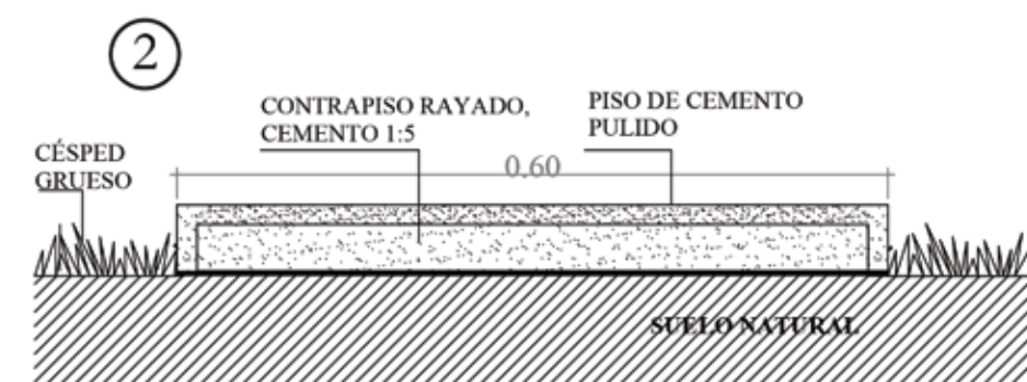
DETALLE DE PLACAS DE HORMIGO - CAMINERAS ESC 1/20
