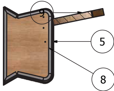
Corte N-N ( 1: 20 )
