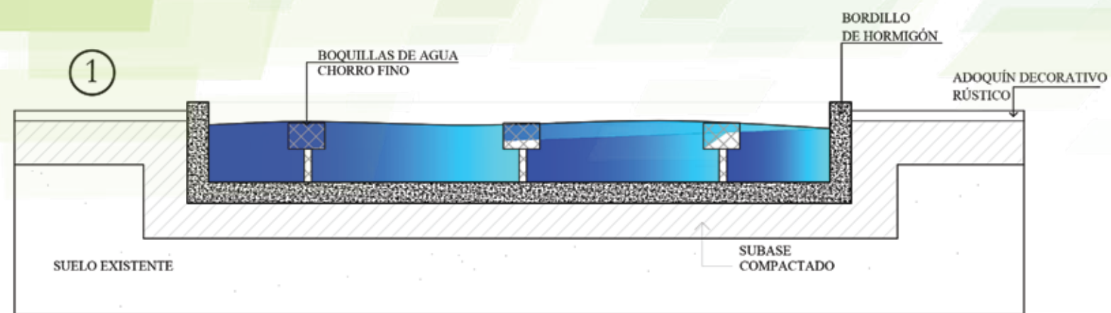
DETALLE DE FUENTE TIPO PILETA ESC 1/50
