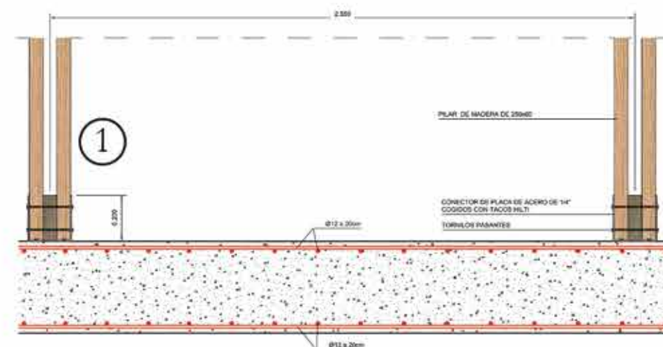
DETALLE DE ANCLAJE DE PERGOLA (EJE X) ESCALA: 1/20
