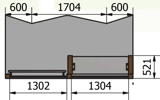
VISTA INFERIOR
