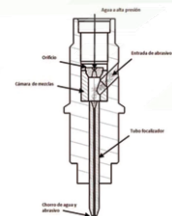
DETALLE BOQUILLA DE AGUA ESC 1/10
