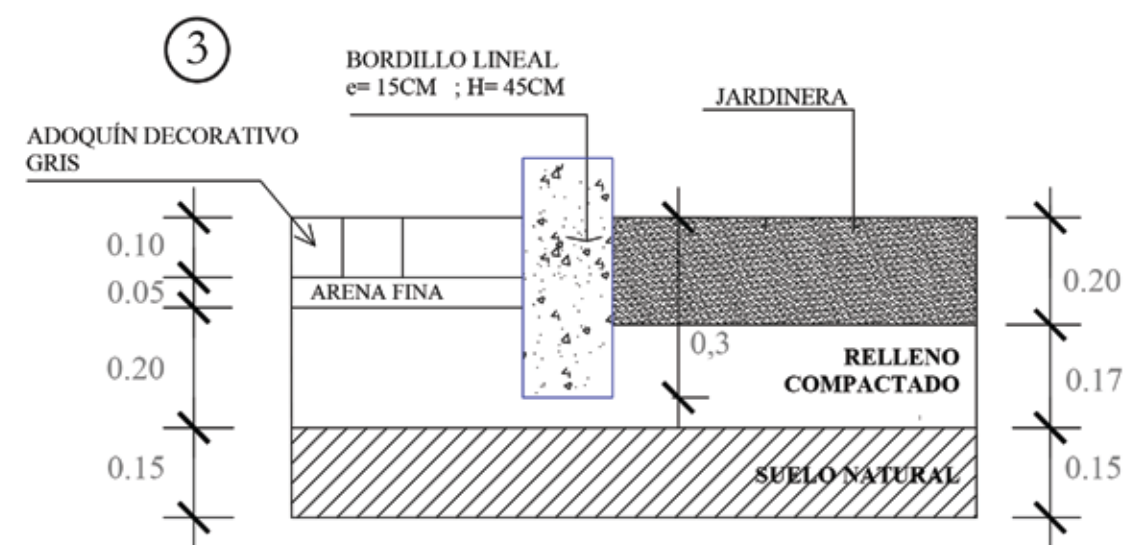
DETALLE ENTRE ADOQUÍN Y JARDINERA ESC 1/10
