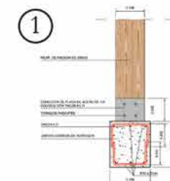
DETALLE DE ANCLAJE DE PERGOLA (EJE Y) ESCALA: 1/20
