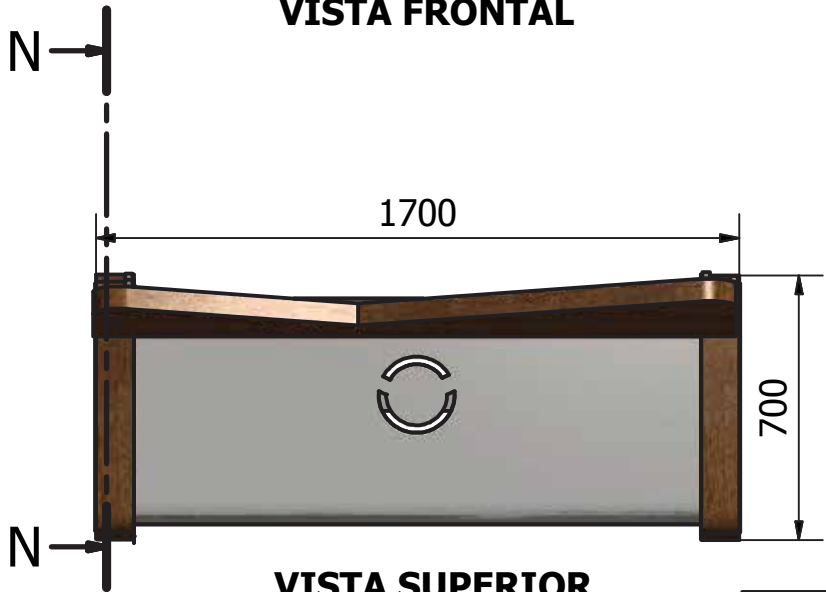
VISTA SUPERIOR
