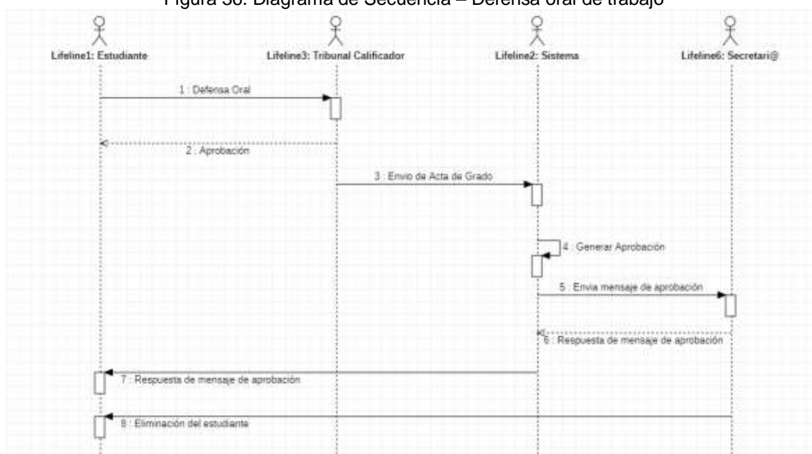
Figura 36. Diagrama de Secuencia – Defensa oral de trabajo
