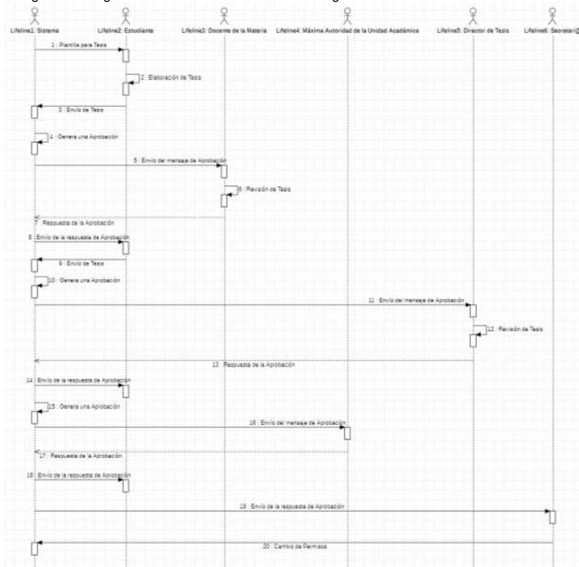
Figura 29. Diagrama de Secuencia – Proceso de integración curricular/Seminario de titulación
