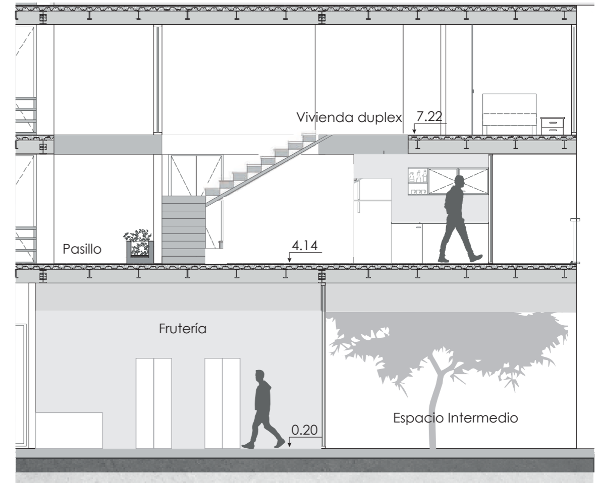
CORTE A-A BLOQUE C
