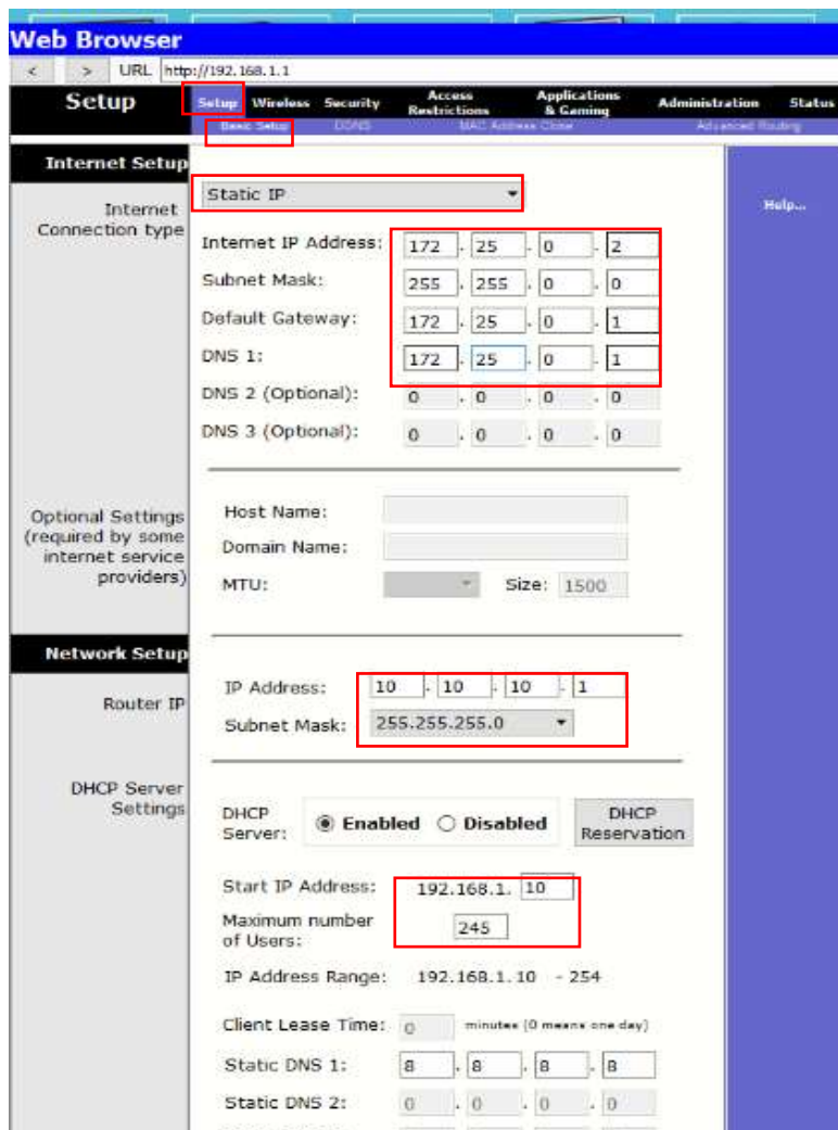
Figura 23 Pestaña principal de Router
