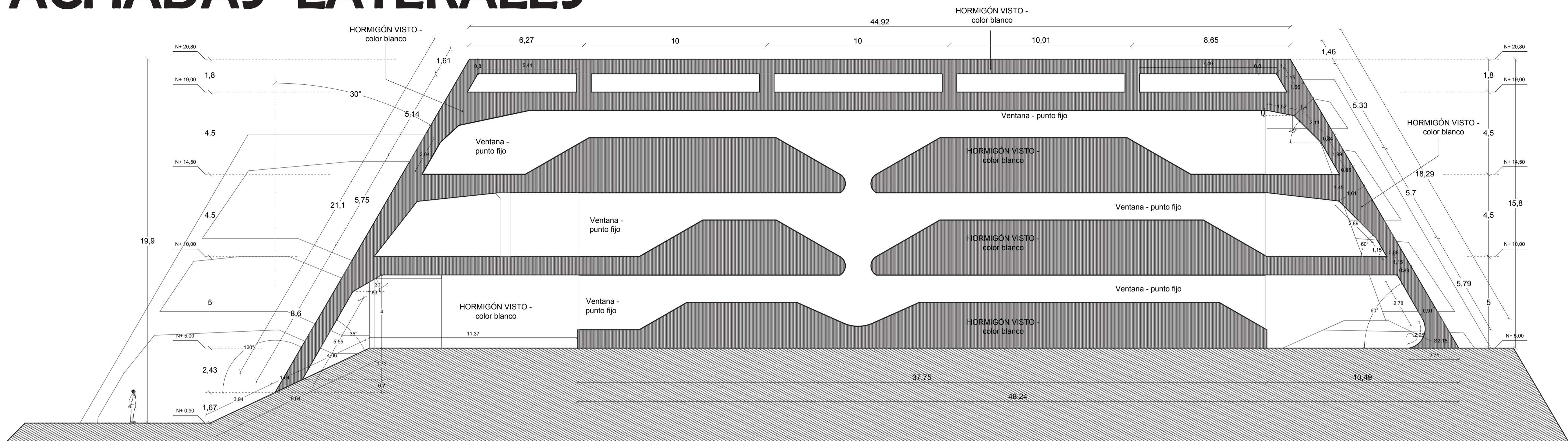
FACHADA LATERAL DERECHA escala - 1:120
