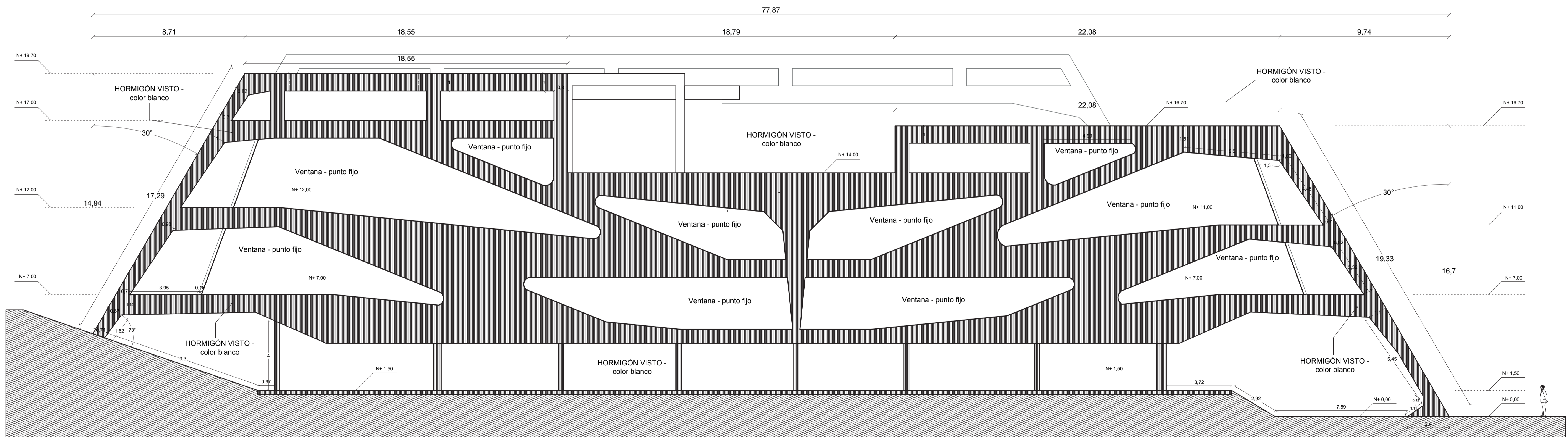
FACHADA LATERAL IZQUIERDA escala - 1:120
