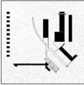
Bloque 4. Corte A-A' E. 1:100
