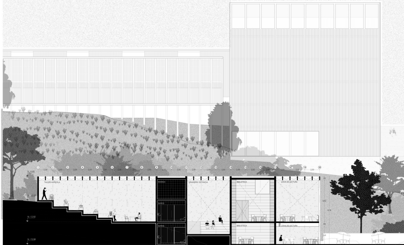
Bloque 5. Corte A-A' E. 1:100
