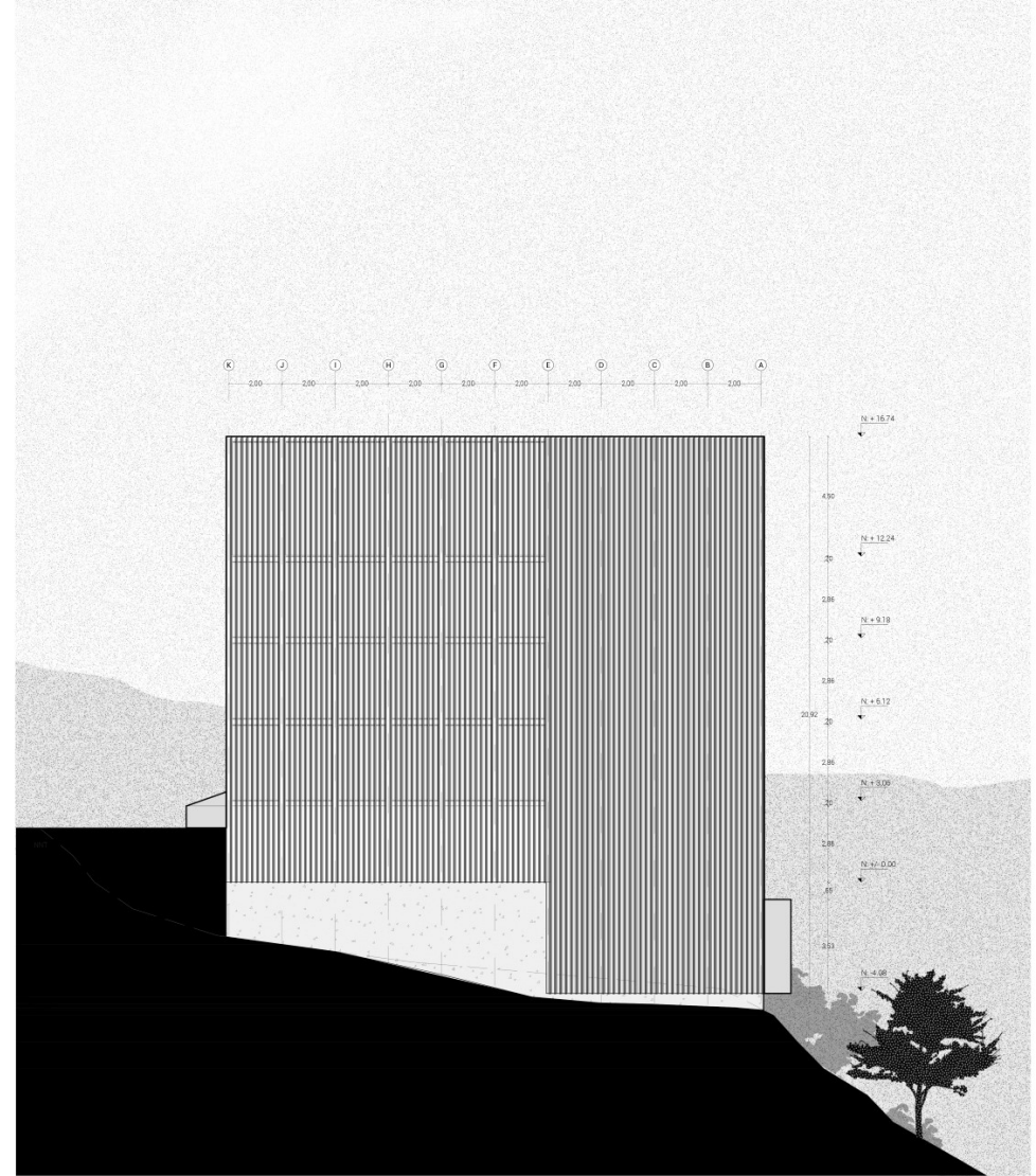
Bloque 1, Fachada Lateral 2 E. 1:100
