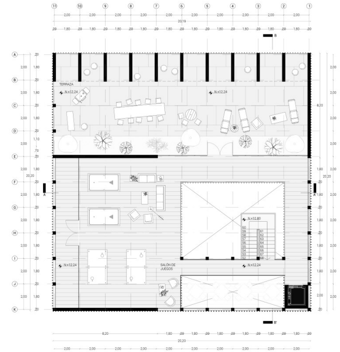
Bloque 1. Planta N: +12.24 E. 1:100
