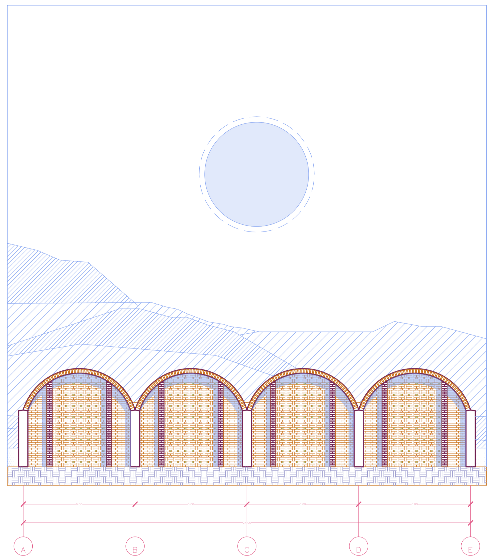
FACHADA FRONTAL
