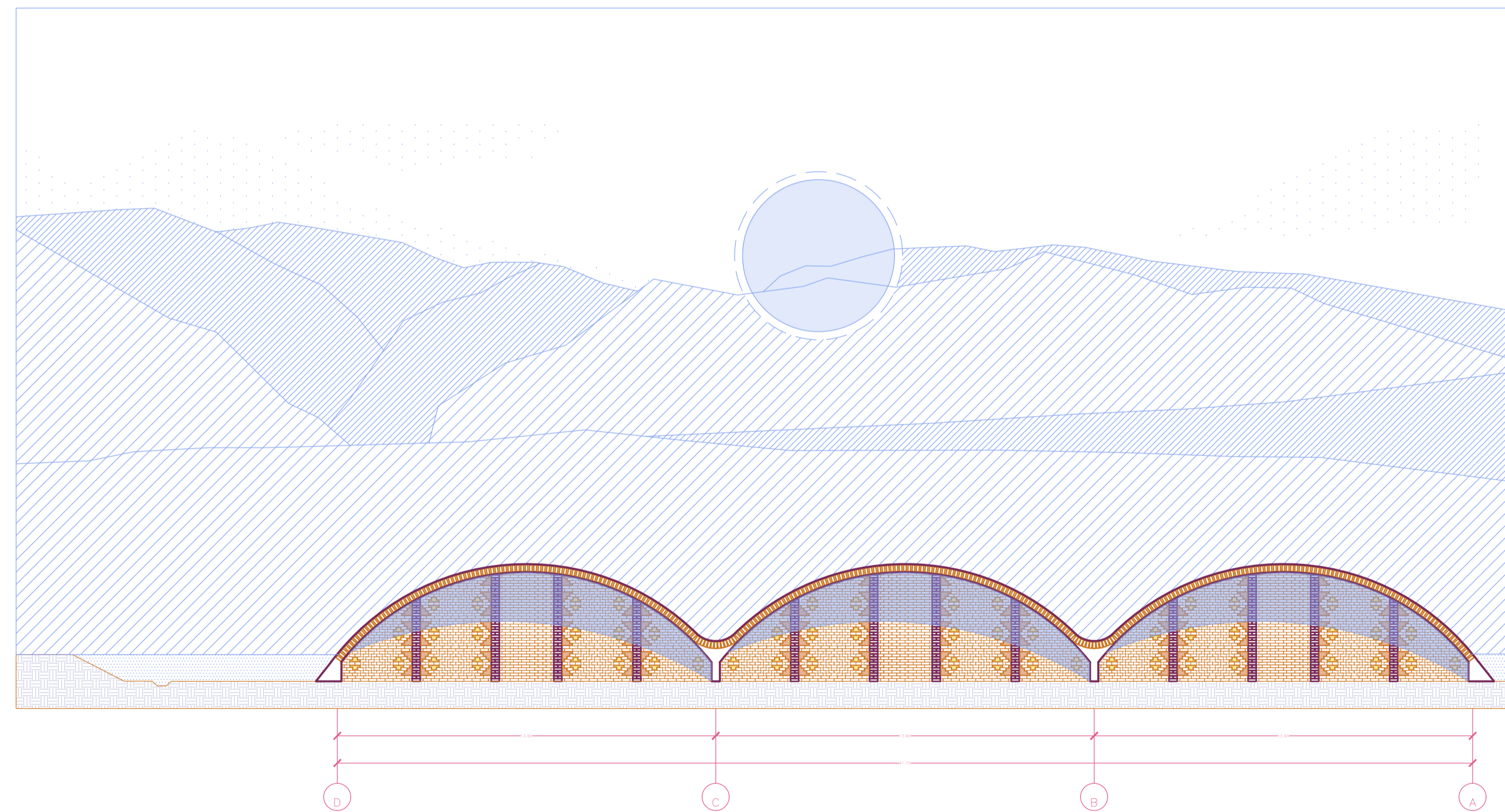
FACHADA POSTERIOR
