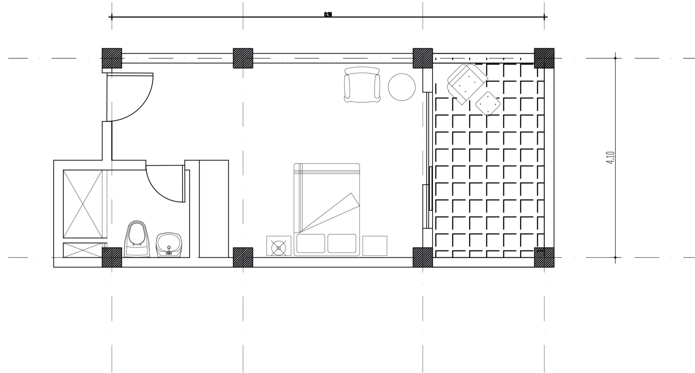
Planta Tipo #2 esc: 1:200
