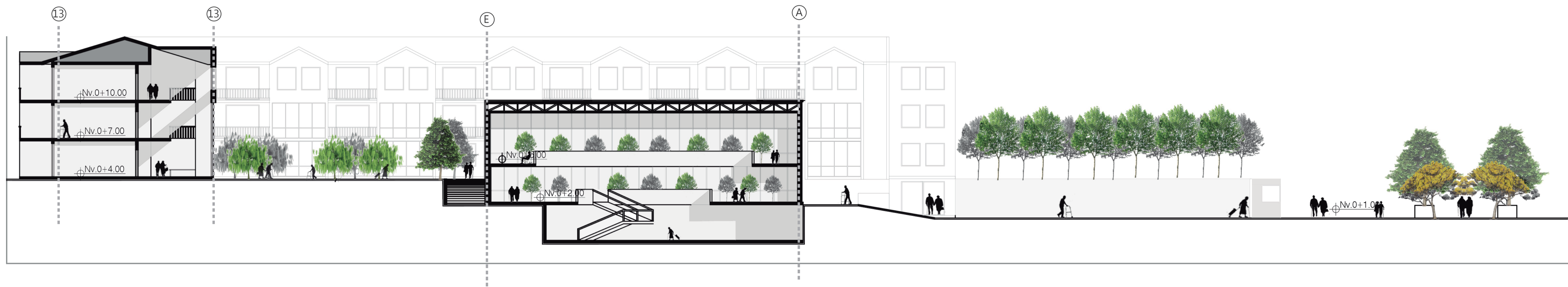
Corte A - A' esc: 1:250
