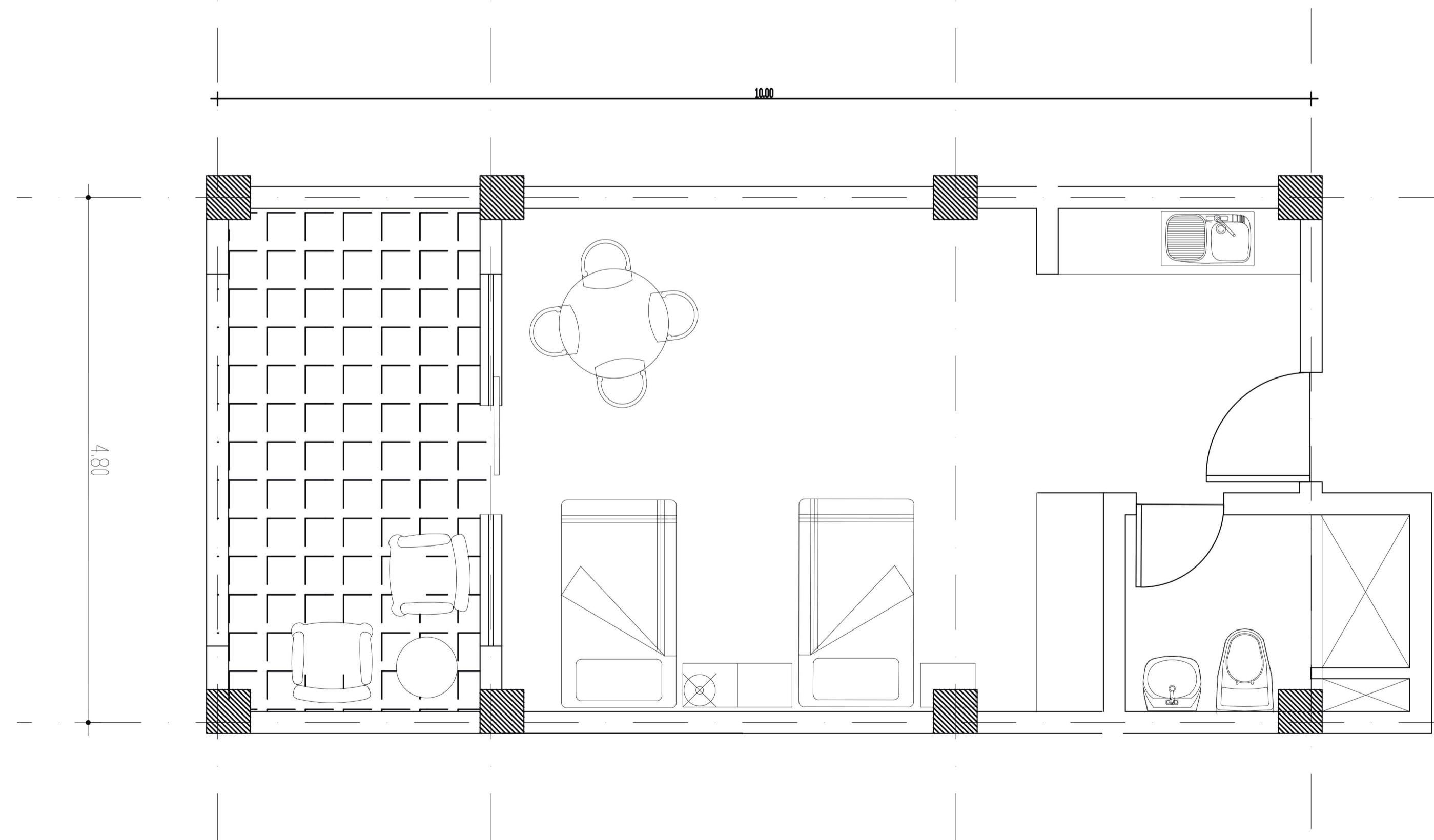
Planta Tipo #2 esc: 1:200
