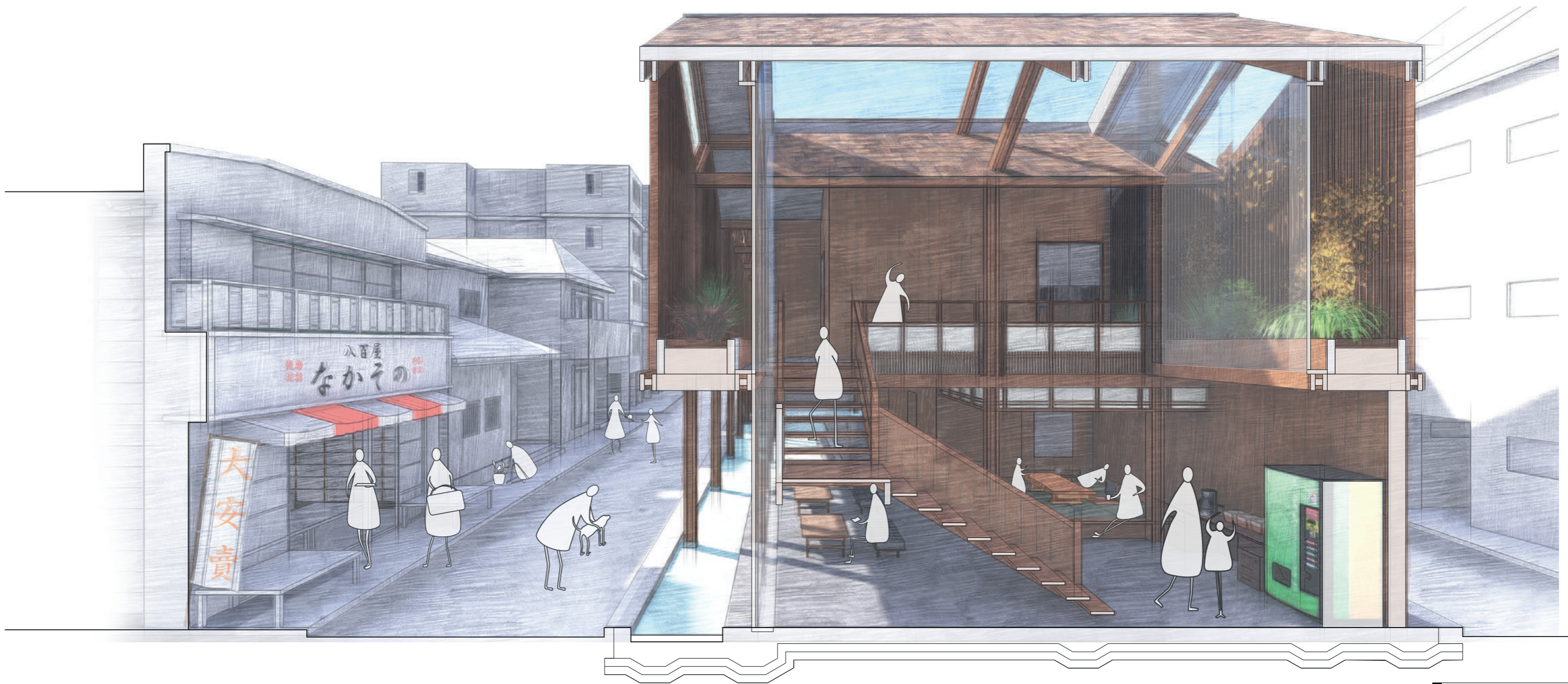
CORTE PERSPECTICO TIPO I
