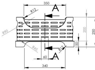
SECCIÓN A-A
