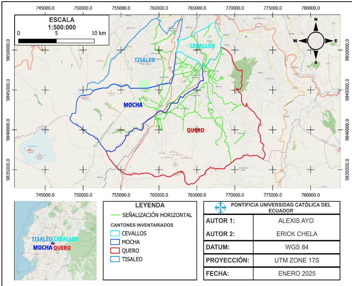
Figura N° 61. Mapa de la señalización horizontal existente en la red vial 2024 de los cantones Cevallos, Quero, Tisaleo y Mocha
