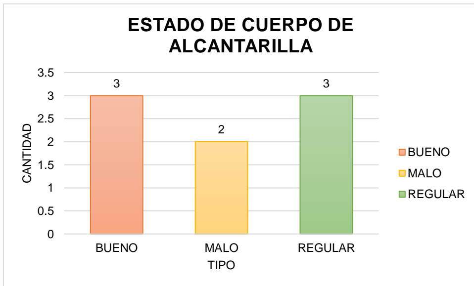
Figura N° 44. Atributo de estado de cuerpo de alcantarilla - cantón Cevallos
