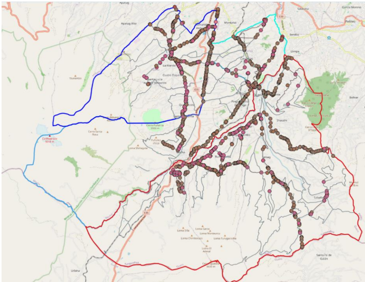
Figura N° 3. Extracción de capas para los cantones Cevallos, Quero, Tisaleo y Mocha desde la Geodatabase de la provincia de Tungurahua (Elaboración propia)
