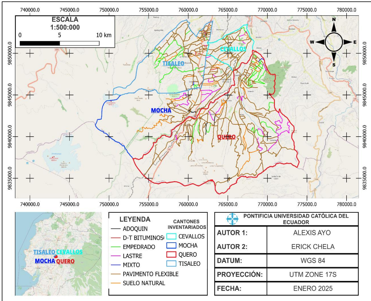
Figura N° 59. Mapa de tipo de superficie de rodadura de la red vial 2024 de los cantones Cevallos, Quero, Tisaleo y Mocha
