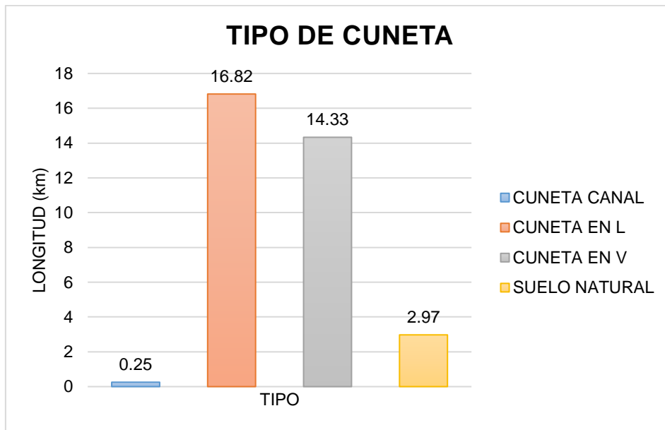
Figura N° 30. Atributo de tipo de cuneta - cantón Tisaleo
