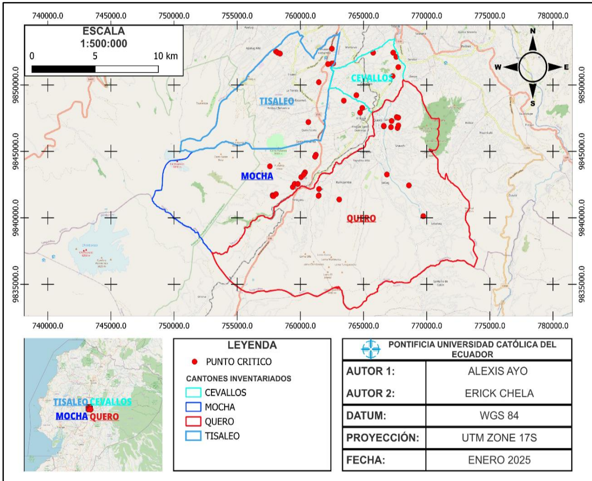
Figura N° 65. Mapa de puntos críticos existentes en la red vial 2024 de los cantones Cevallos, Quero, Tisaleo y Mocha
