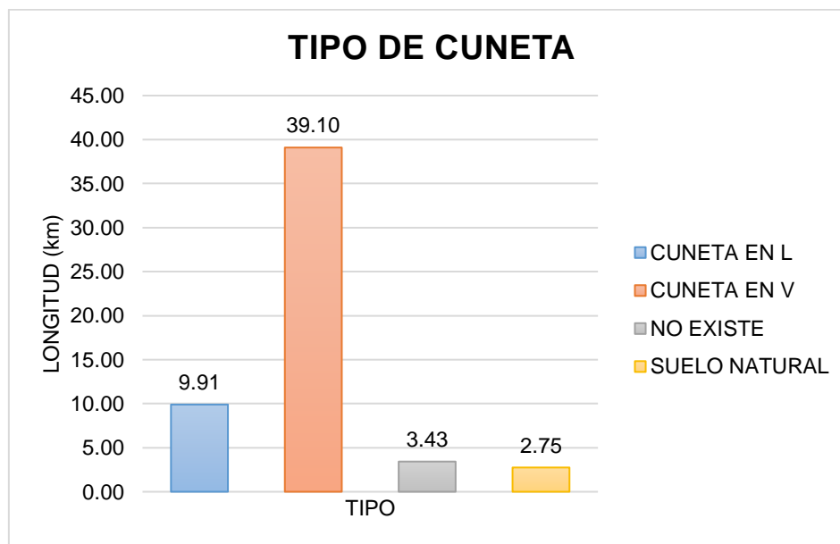
Figura N° 28. Atributo de tipo de cuneta - cantón Quero
