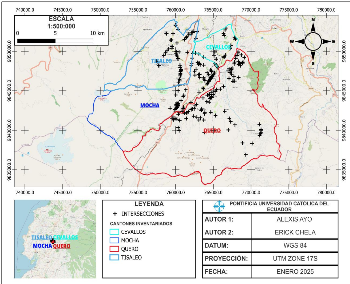
Figura N° 67. Mapa de intersecciones existentes en la red vial 2024 de los cantones Cevallos, Quero, Tisaleo y Mocha
