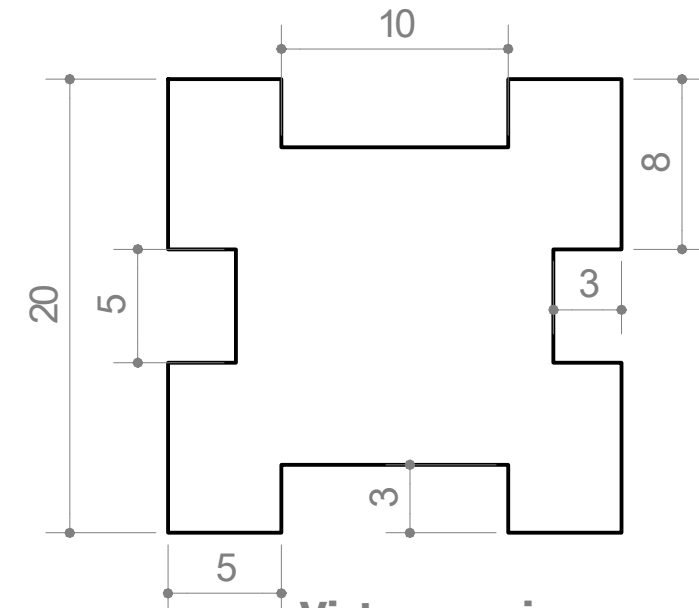
Vista superior
